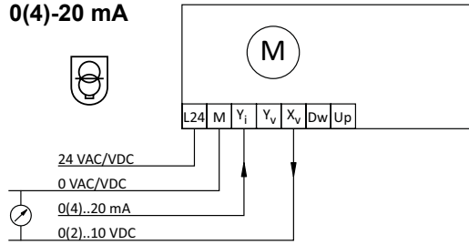
0(4)-20 mA
