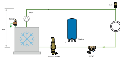
Hladilni sistem
