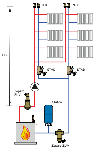
Sistem ogrevanja
