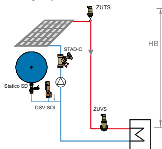
Solarno ogrevanja
