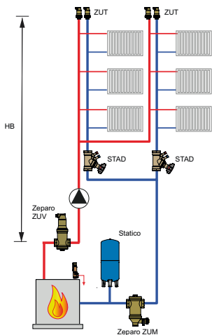
Circuit încălzire
