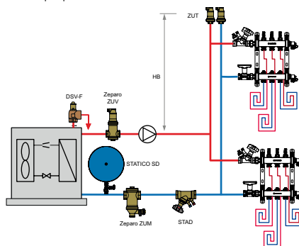
Circuit cu pompă de căldură
