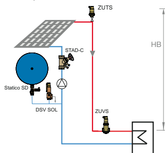
Circuit cu panouri solare
