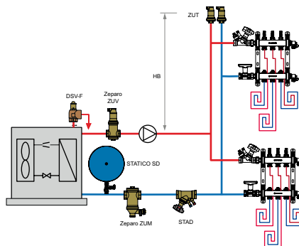
Sistema con Bomba de Calor
