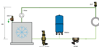
Sistema de refrigeración
