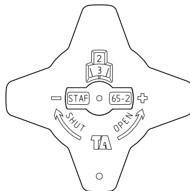
Fig. 2 Válvula ajustada en la posición 2.3
