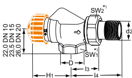
Escuadra inversa con longitud reducida. Latón. No es adecuado para el montaje de las tuberías multicapa de compresión.
