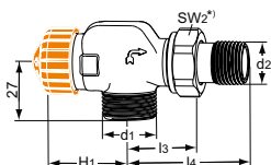
Escuadra inversa con rosca macho G3/4
