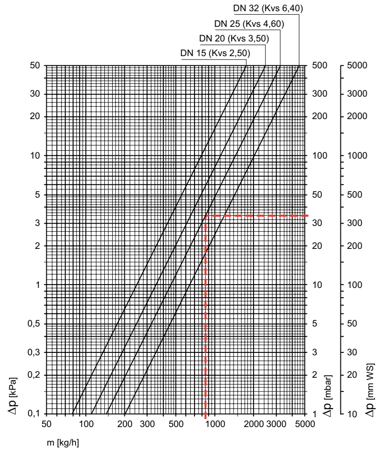
Diagramm, Dreiwege-Mischventil, k_{vs} -Werte
