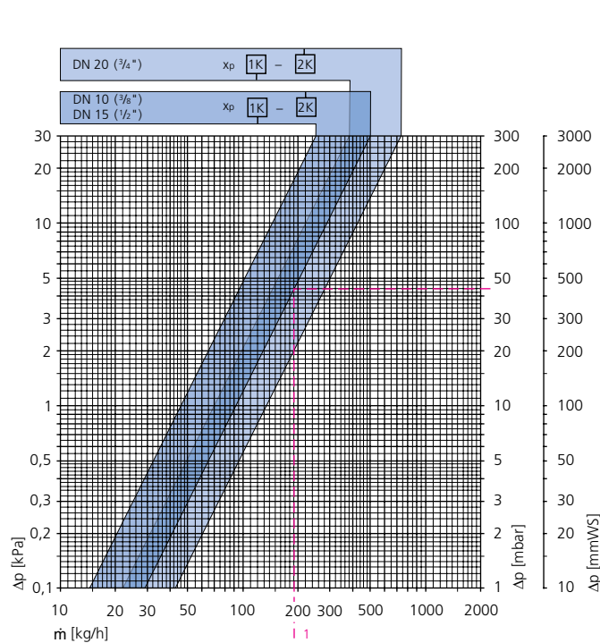
Diagram DN 10 (3/8") til DN 20 (3/4"), radiatorventil med termostat
