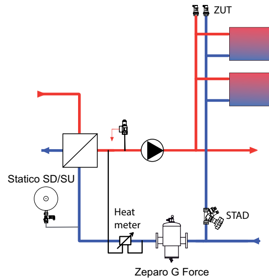
System met warmtewisselaar
