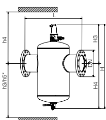
Vuilafscheider
